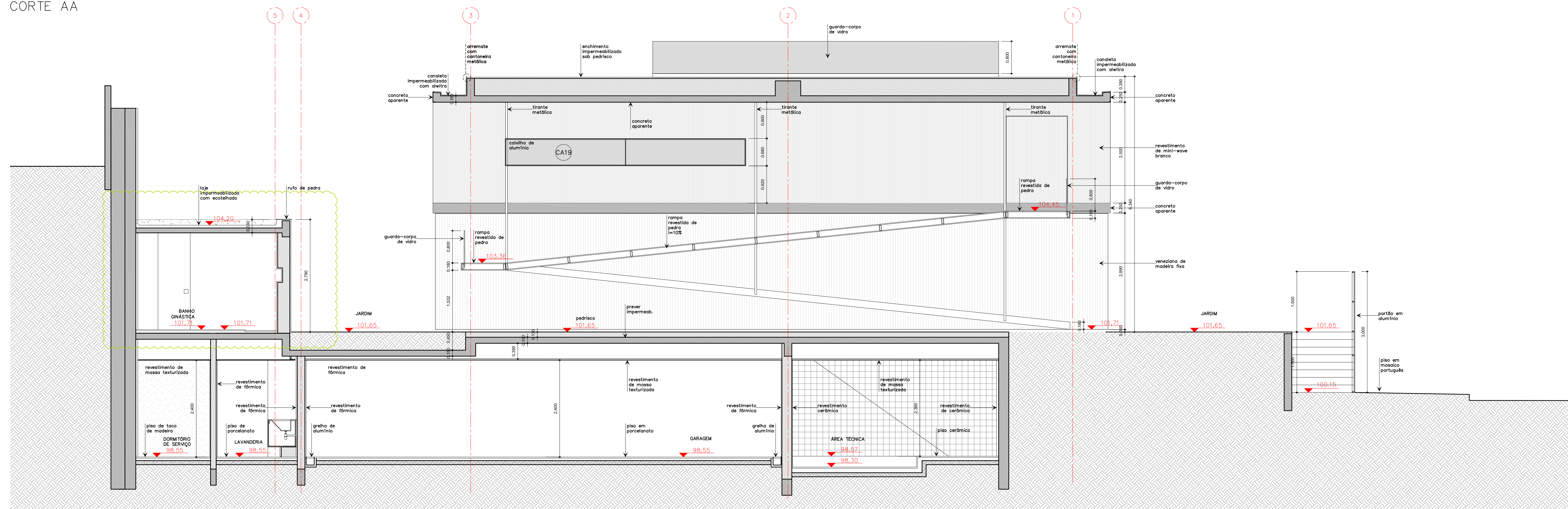
CORTE BB
