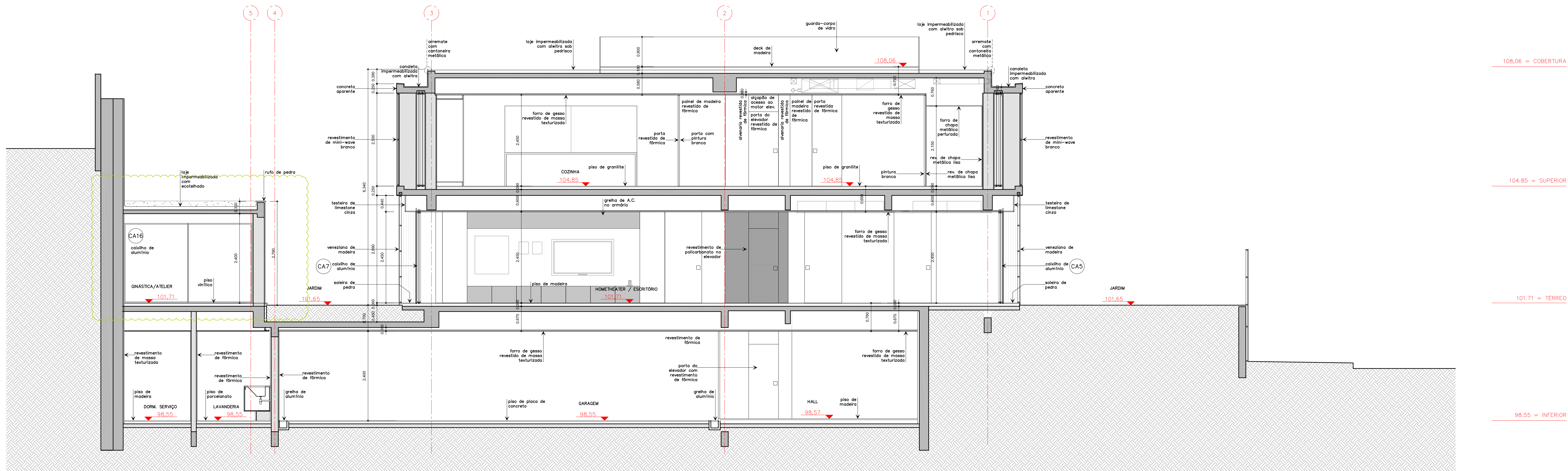
CORTE DD
